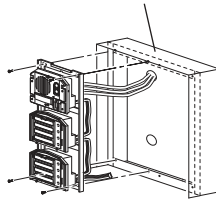
Påbygningsboks med regnskærm GT 203HB
