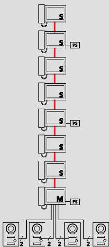
Seriekabling
