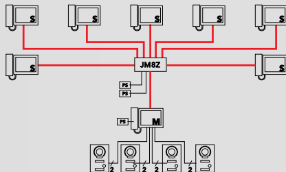
Stjerne kabling
